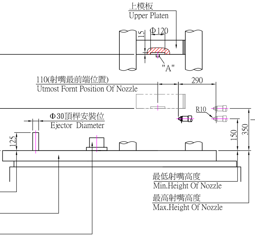
開合模規格示意圖(Clamping Unit Diagram)
