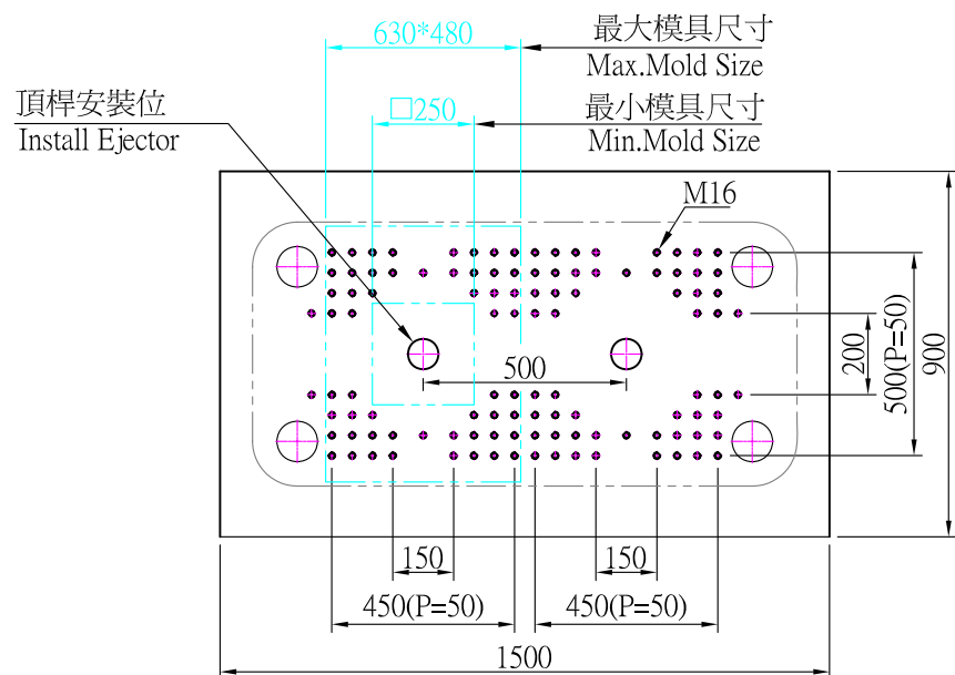
下模板(Bottom Platen)
