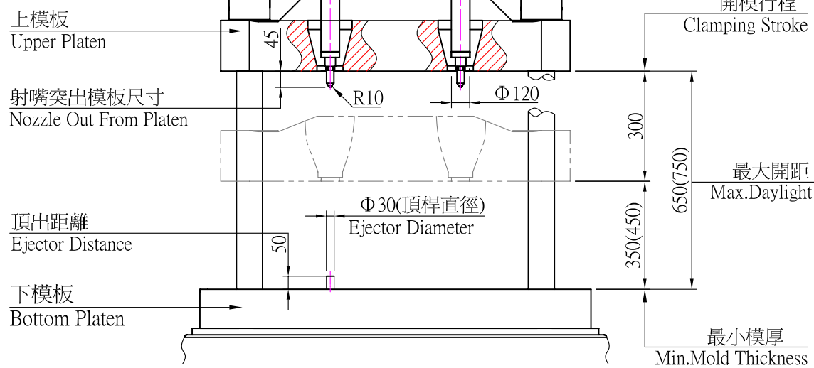
開合模規格示意圖(Clamping Unit Diagram)
