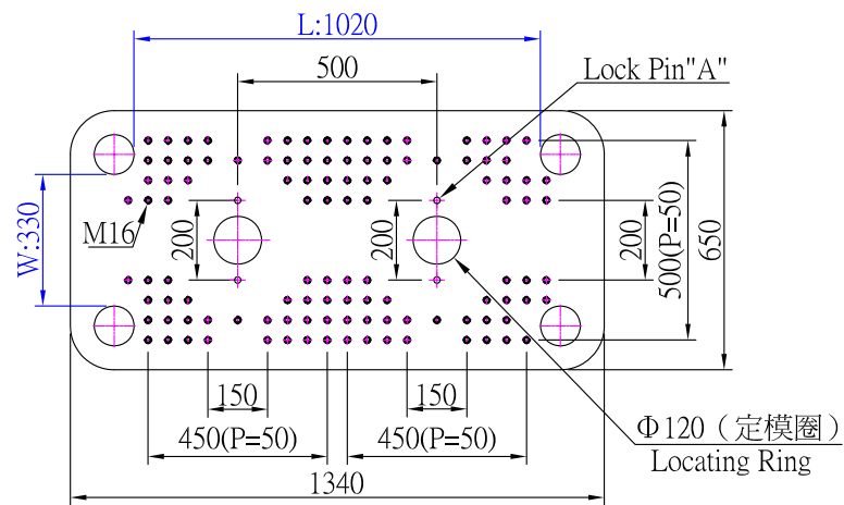
上模板(Upper Platen)
