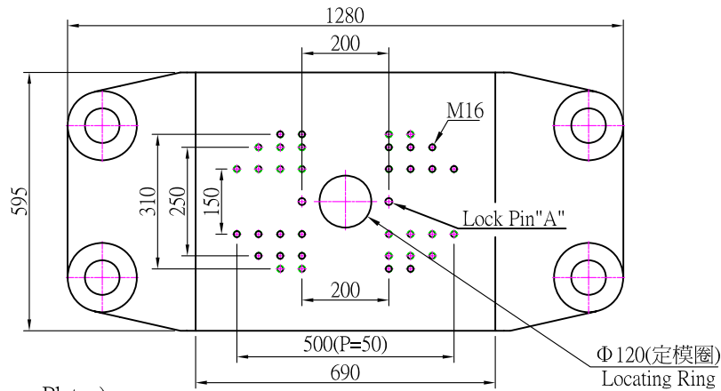
上模板(Upper Platen)
