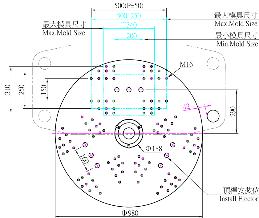
轉盤模板(Rotary Platen)
