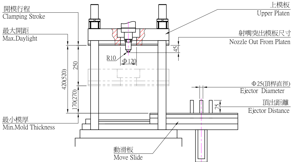
開合模規格示意圖(Clamping Unit Diagram)
