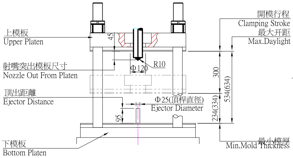
開合模規格示意圖(Clamping Unit Diagram)
