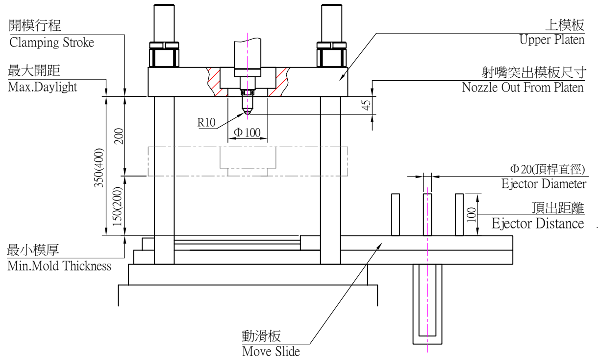
開合模规格示意图(Clamping Unit Diagram)
