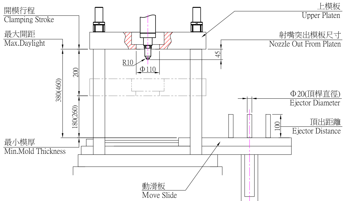
開合模規格示意圖(Clamping Unit Diagram)
