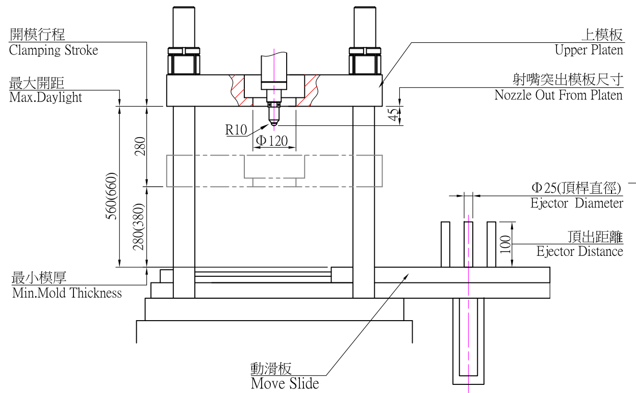
開合模規格示意圖(Clamping Unit Diagram)
