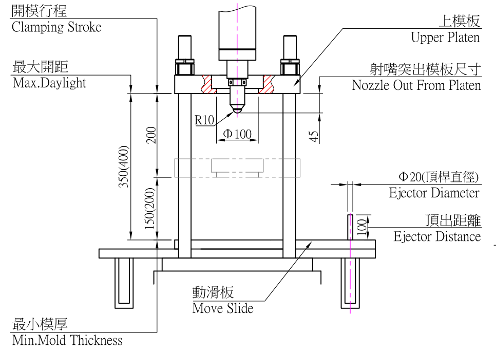
開合模規格示意圖(Clamping Unit Diagram)
