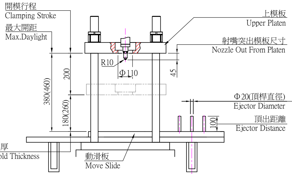
開合模規格示意圖(Clamping Unit Diagram)
