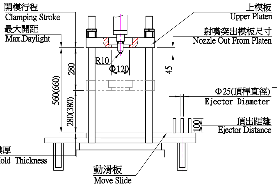
開合模規格示意圖(Clamping Unit Diagram)
