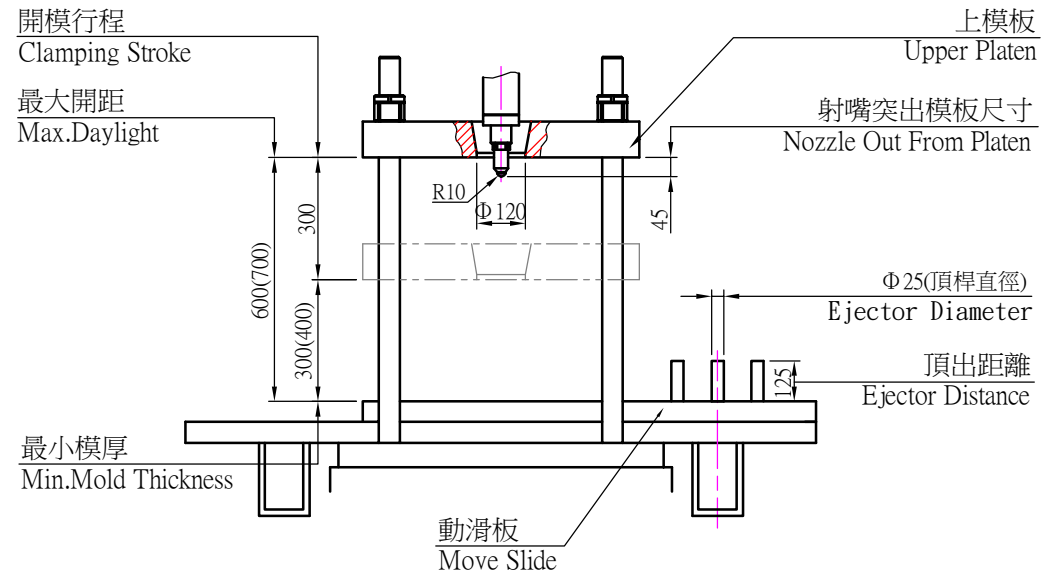
開合模規格示意圖(Clamping Unit Diagram)
