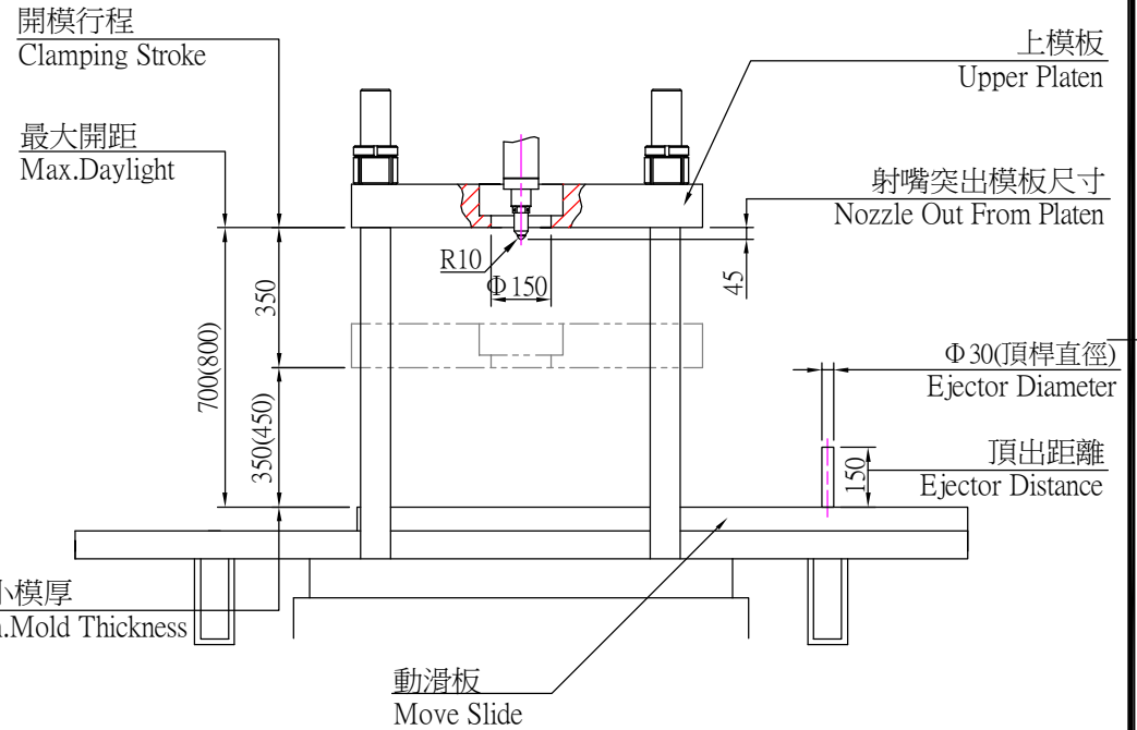
開合模規格示意圖(Clamping Unit Diagram)
