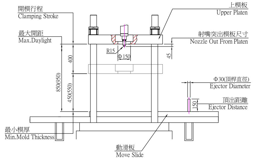
開合模規格示意圖(Clamping Unit Diagram)
